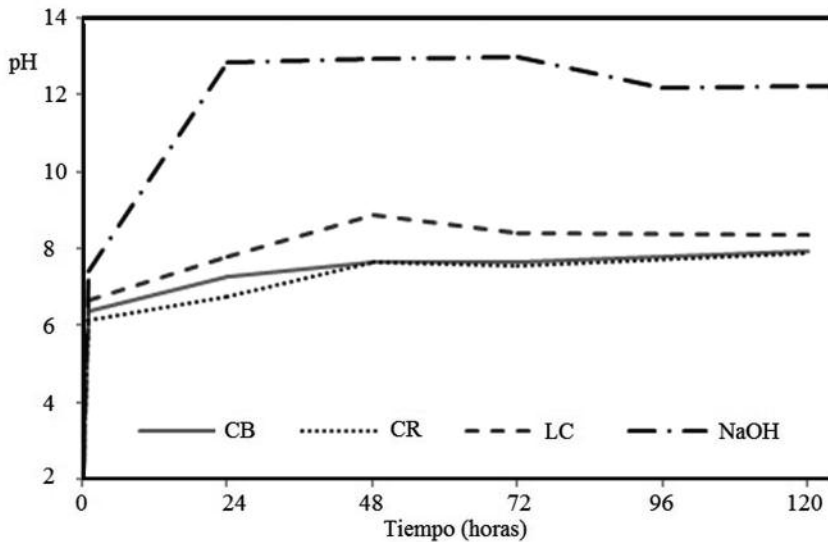
Fig. 1.- Evolución del pH a lo largo del tratamiento de la muestra de AMD de la corta de San Telmo con los reactivos neutralizantes.
