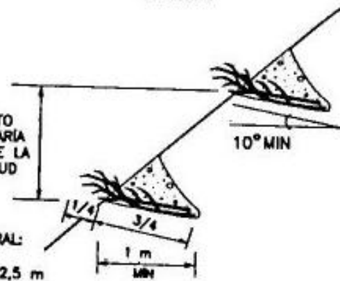
ALZADO A-A'
