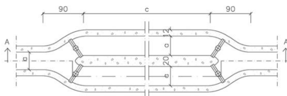
Ilustraciones 5 y 6. Plano del desarenador desengrasador
