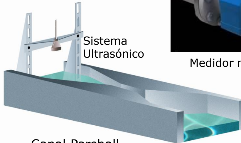
Canal Parshall
