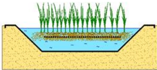
Sistemas FMF (Filtros Macrofitas en Flotación) y FHS (Filtros de Halofitas Sumergido)
