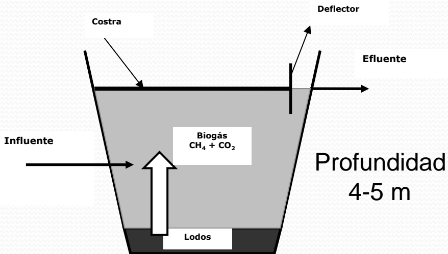
Laguna anaerobia
