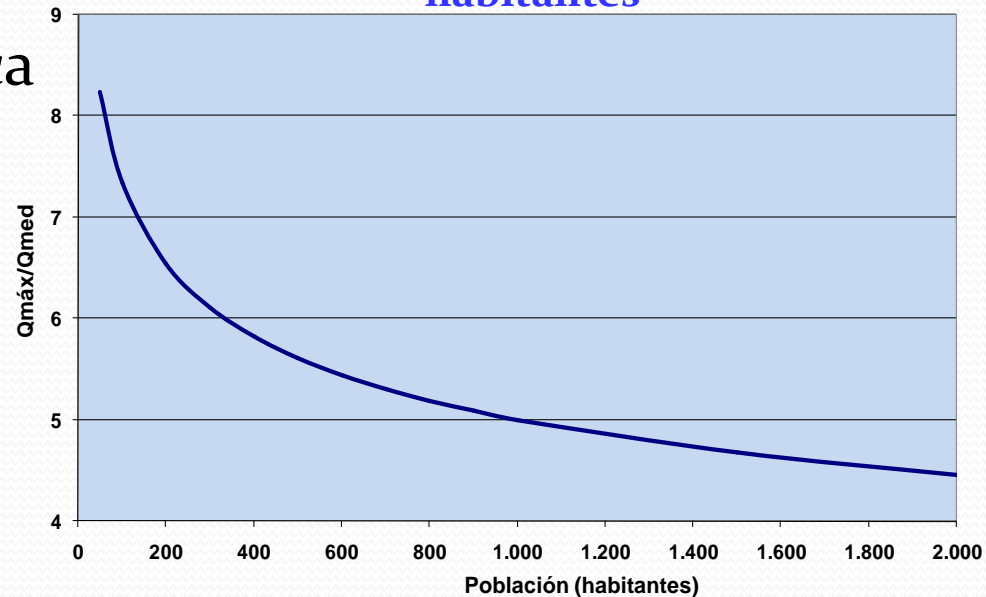
Relación entre Q_{\max}/Q_{\text{med}} y nº de habitantes
