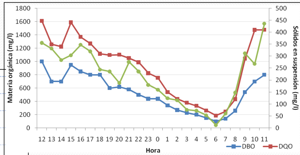
Evolución diaria de las concentraciones (DBO, DQO y SS)
